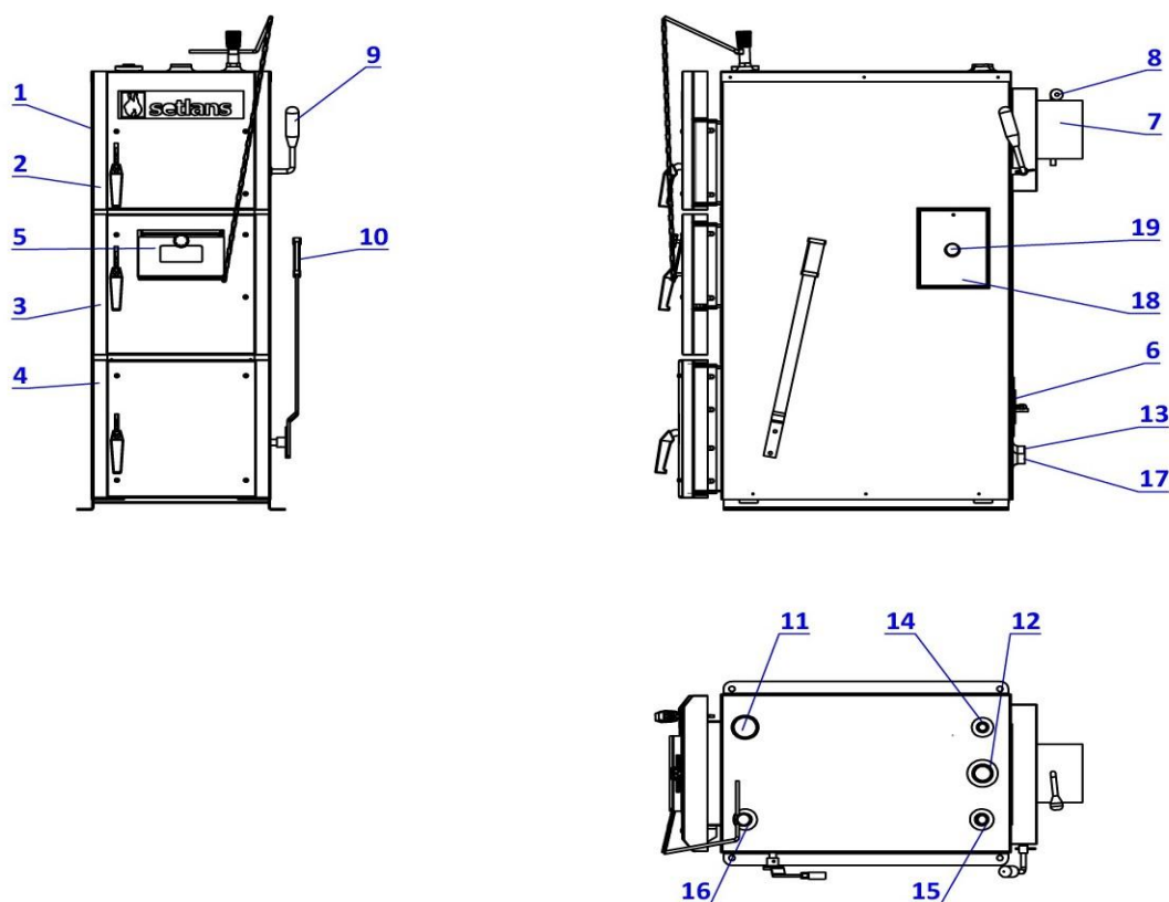
Rys. 1 Budowa kotła Setlans Selvan
