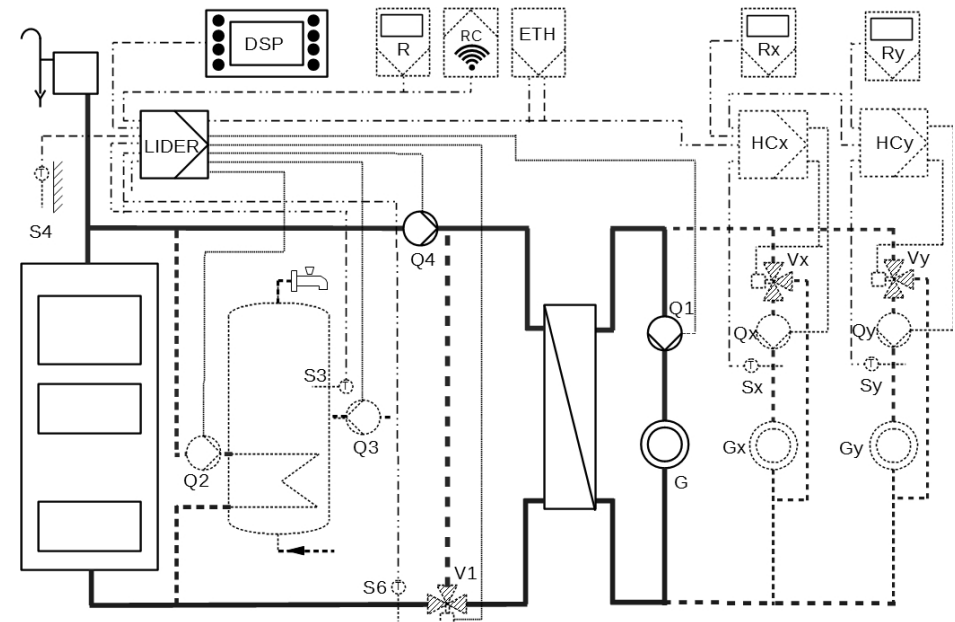
Schemat podłączeń:
